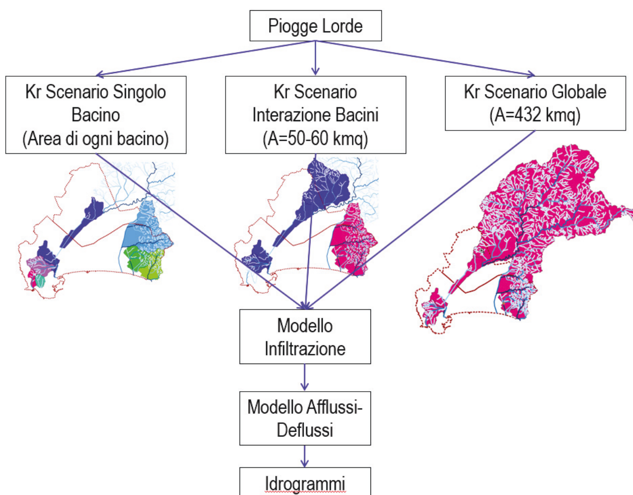
Figura 4-1: Schema logico della modellistica idrologica
